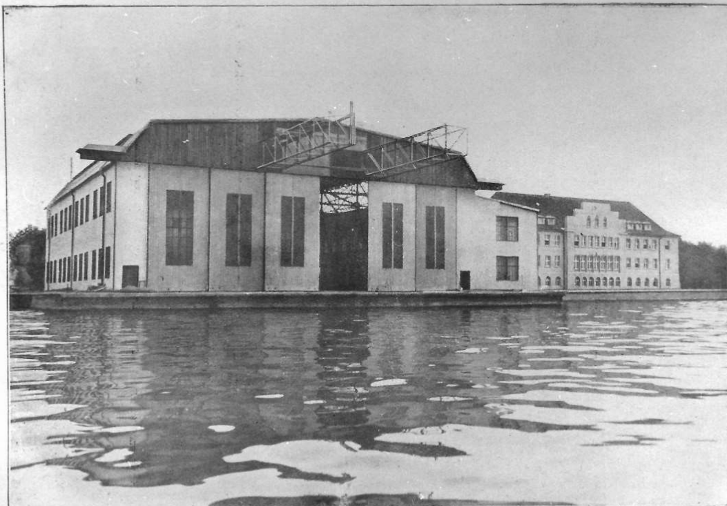
Bootsbau-Halle mit Krangerüst. Seeseite.
